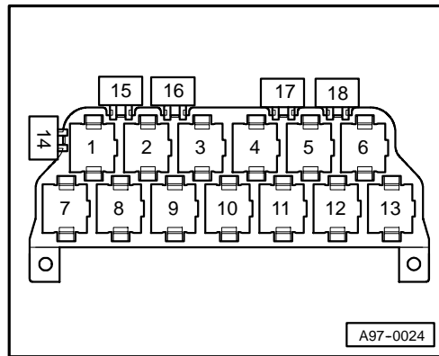
Porte-relais à 13 raccords (sous le vide-poches côté conducteur)
