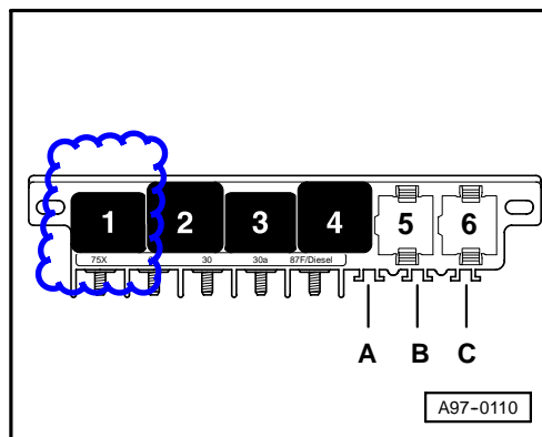
Petite centrale électrique (sous le vide-poches, côté conducteur)
