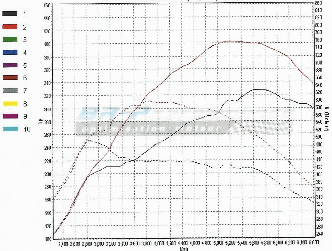
Puissance-max Puissance Moteur (corr.) / Couple (corr.) / Vitesse
